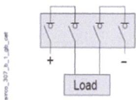
4极 (1000VDC): 两极串联为正负极
