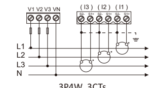
3P4W 3CTs
